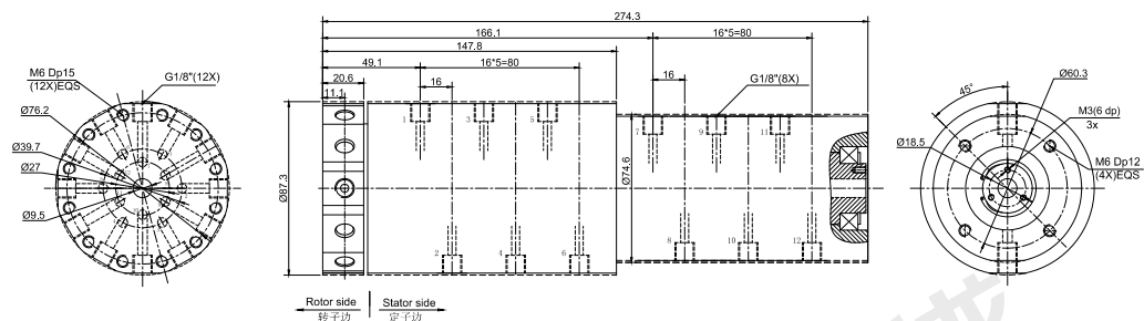
MCGP161 (紧凑型多功能旋转接头) 尺寸图 16进16出G1/8"牙
